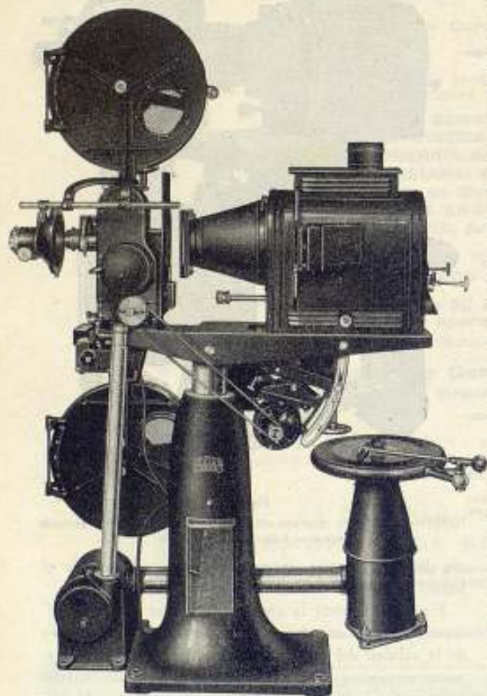
Fig. 2 ERNEMANN II con aparato adicional ZEISS IKON para película sonora. Lado de la transmisión
