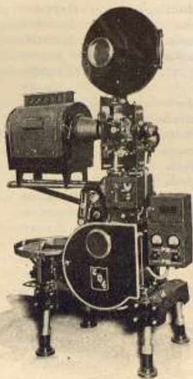
El gran aparato «Super Model», construido a base de circuitos dobles, que da la seguridad al empresario de la imposibilidad de sufrir paro alguno por avería
