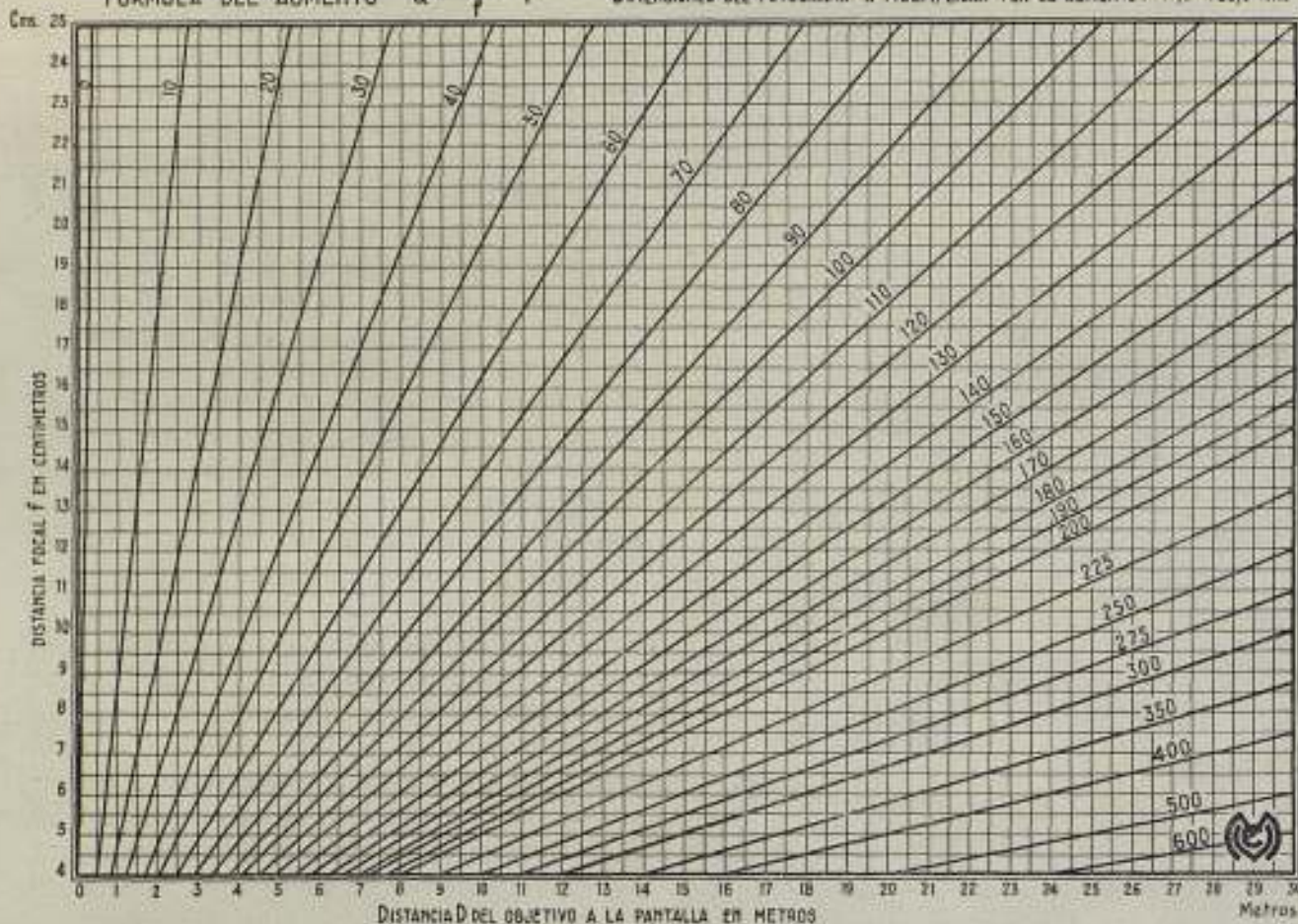
DIAGRAMA PARA DETERMINAR LA AMPLIACION DE LA IMAGEN EN FUNCION DE LA DISTANCIA A LA PANTALLA Y DEL FOCO ÓPTICO
