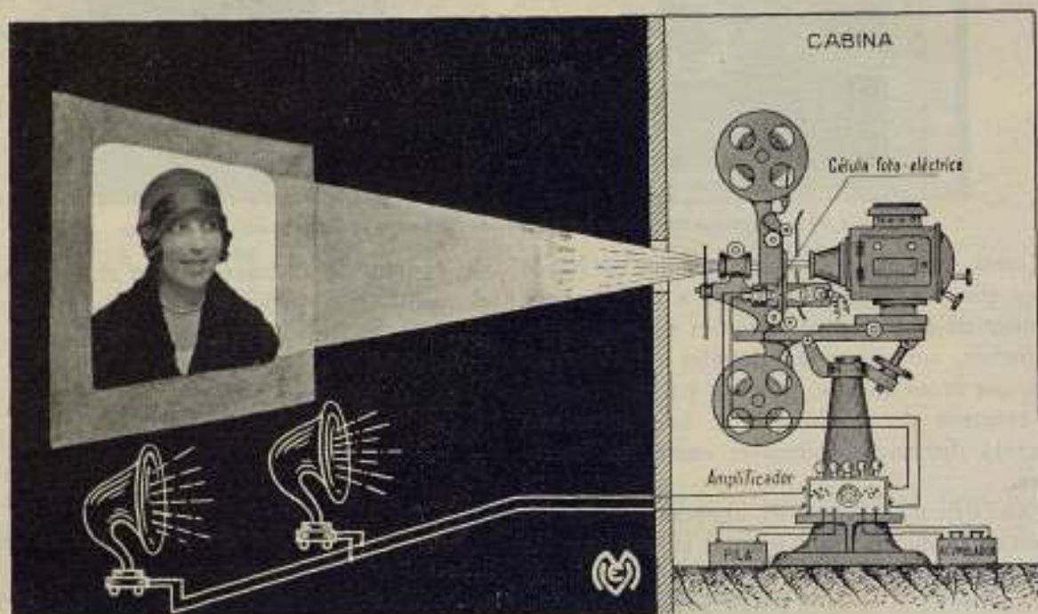
Fig. 6. — Sinópsis de la proyección fonocinematográfica
