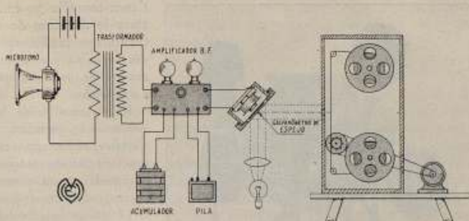
Fig. 7.—Esquema de la impresión sonora en el dispositivo G. P. D.
