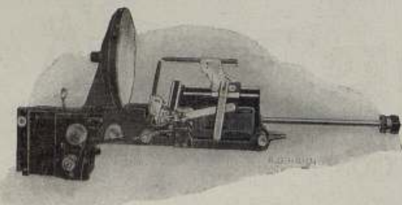
Fig. 1. — Arco de espejo Artisol, con regulador automático.
