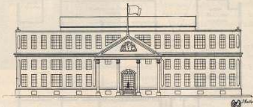
Figura 1.—Fachada principal del estudio. Escala 1:500
