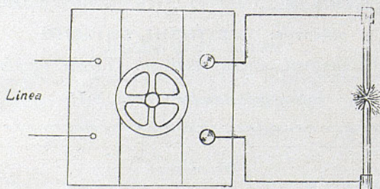
Esquema de conexiones
