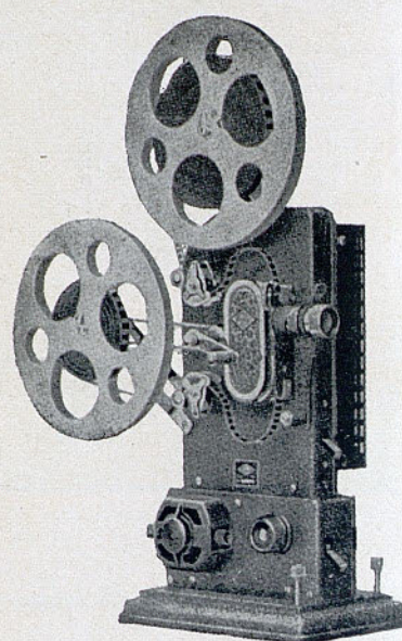
Projector de 9 1/2 o 16 m/m. amb motor, 100 o 200 watts, ideal per a la llar . . . Ptes. 590
