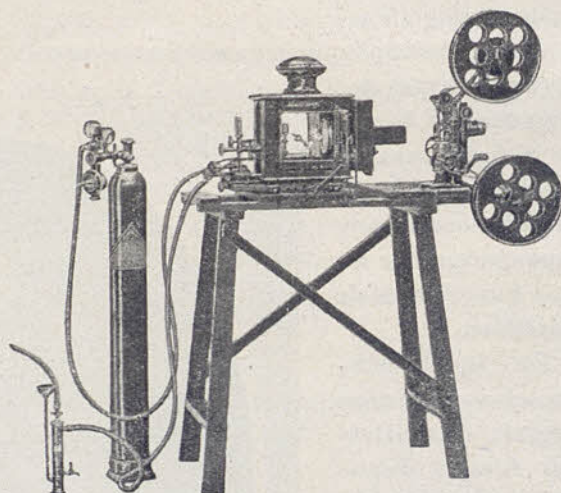
Máquina «Diorama» oxi-aéreo-acetilénica
