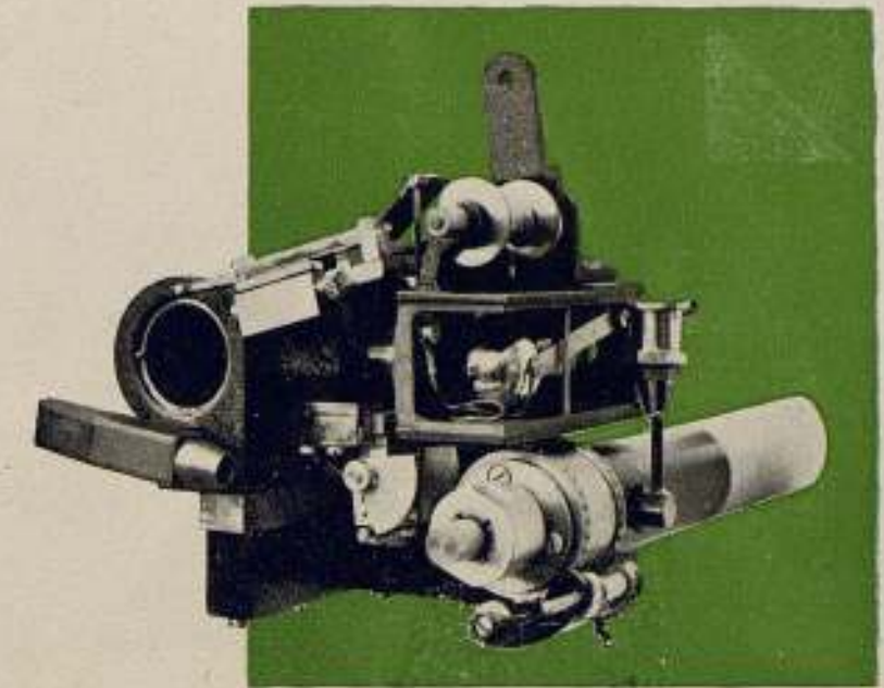
Detalle del equipo Philisonor con la famosa célula fotoeléctrica Philips para la reproducción por banda
