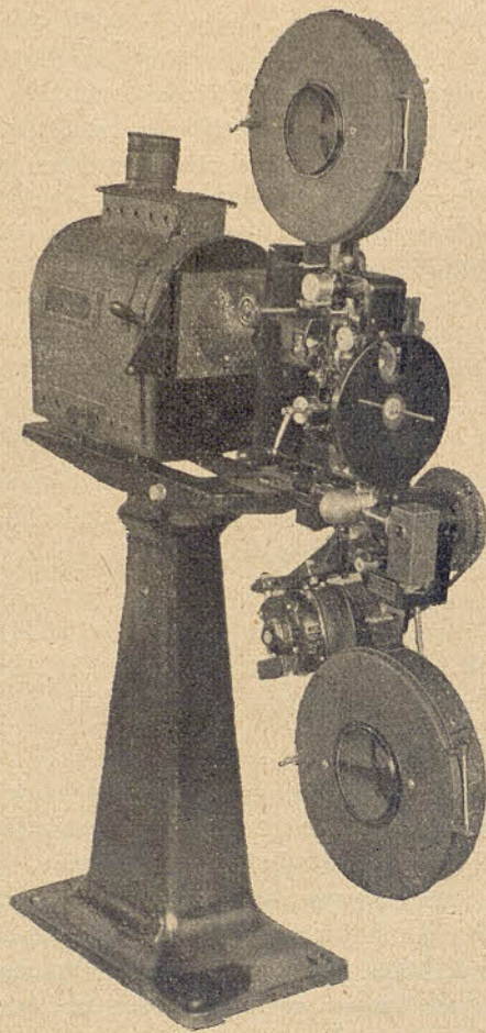
Máquina de proyección O.S.S.A. con caja fotoeléctrica tipo «Record» último modelo. Totalmente fabricada por Orpheo-Sincronic, S. A., Barcelona
