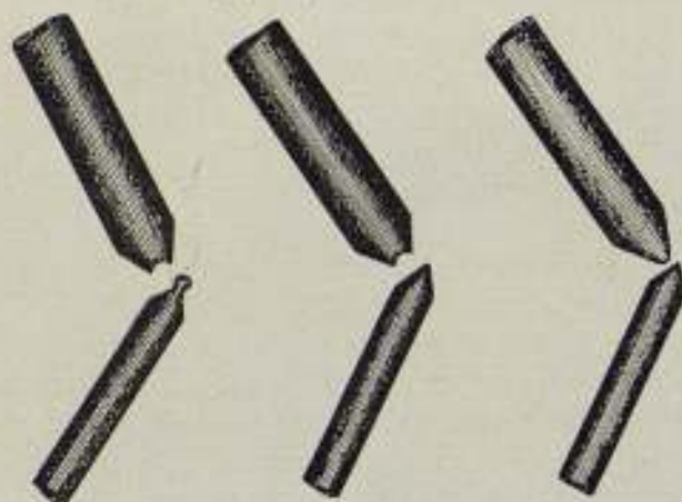
Fig. 3 Fig. 2 Fig. 1 Posición de los carbones en el arco eléctrico
