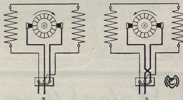
Fig. 5. — Motor-shunt, 3 bornes y manera de invertir el sentido de rotación.
