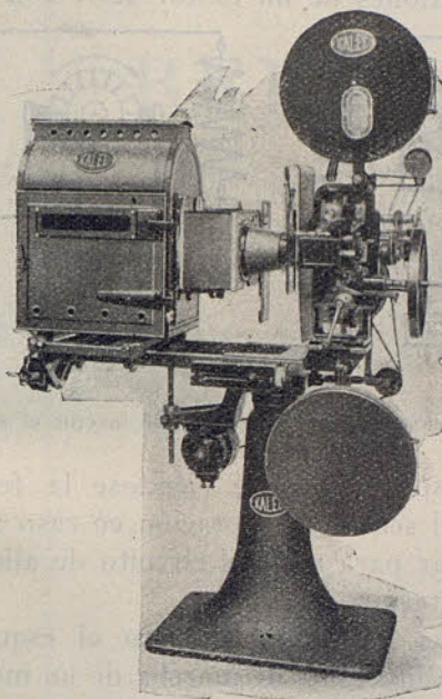
Fig. 1. — Moderno proyector «Kalee», con motor colocado en el chasis.
