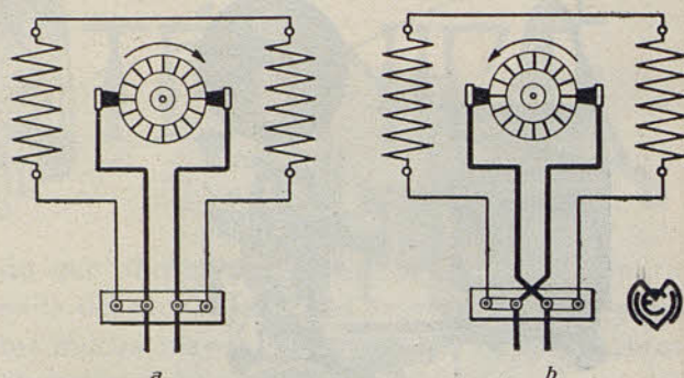
Fig. 4. — Motor-shunt, 4 bornes y manera de invertir el sentido de rotación.
