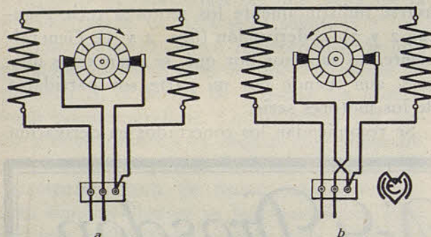
Fig. 3. — Motor-serie, 3 bornes y cambio de su sentido de rotación.
