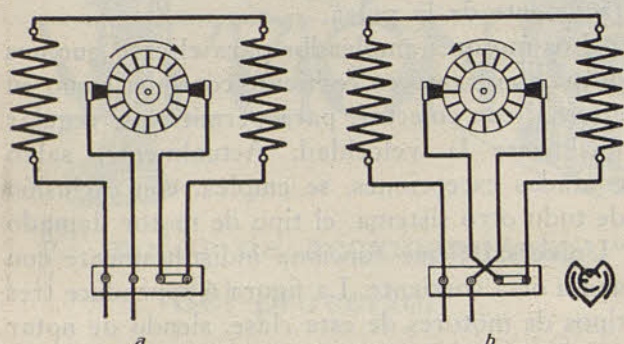
Fig. 2. — Esquema de motor-serie, 4 bornes, con indicación del cambio de sentido de rotación.
