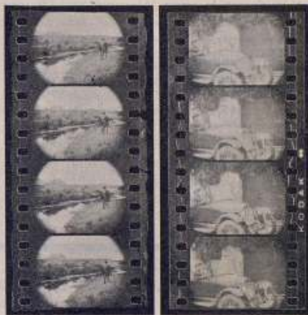
Fig. 4. — Bordes estropeados a causa de pasar el film por balonas combadas.
