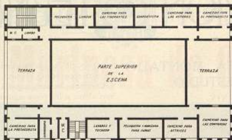
Fig. 9. — Planta del piso tercero. Escala 1:500
