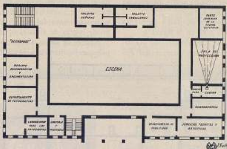
Fig. 8.—Planta del piso segundo. Escala 1:500
