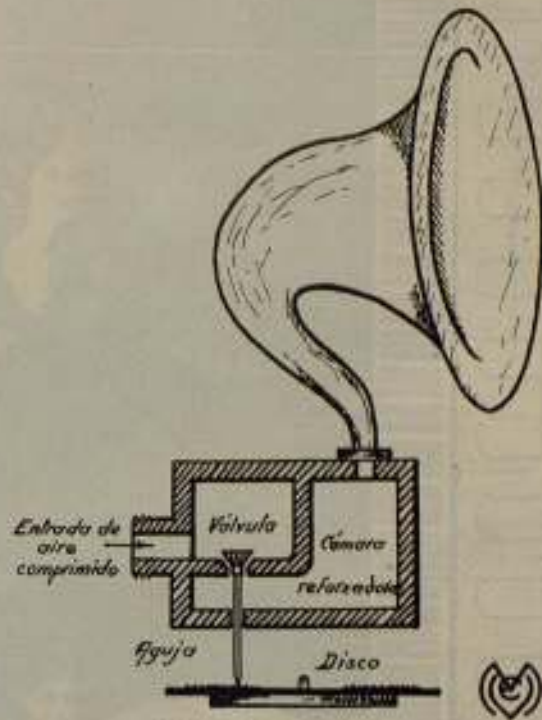
Fig. 1. — Megáfono Gaumont.
