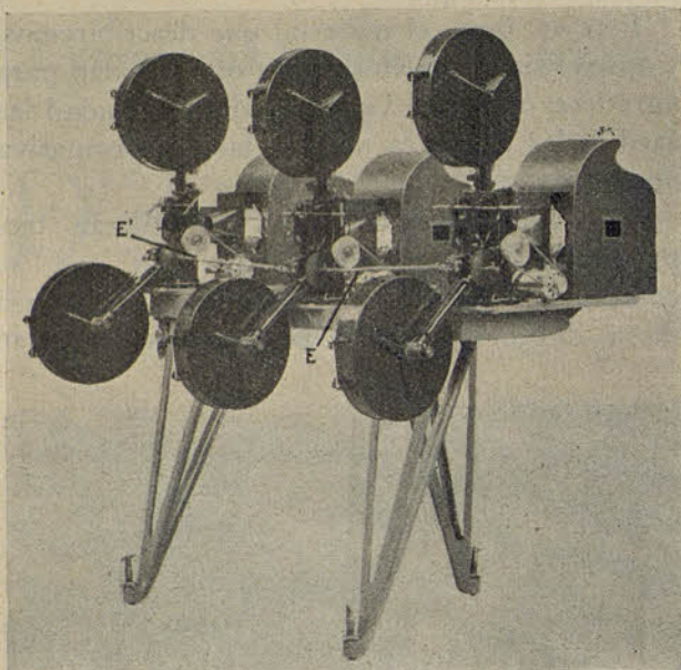
Fig. 7.—Aparato especial Gaumont utilizado en la proyección triptica.
