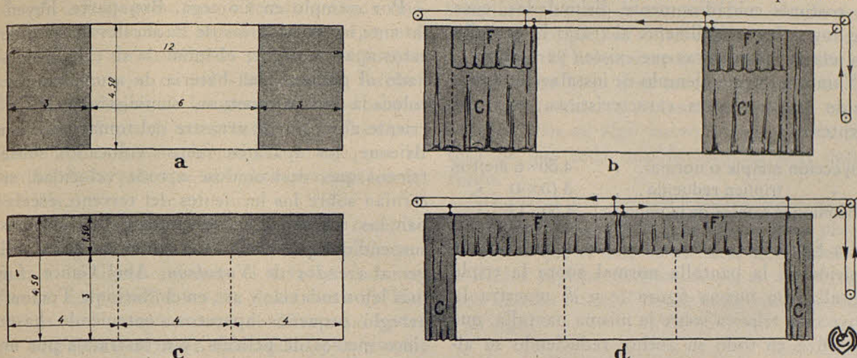
Fig. 9.—Dimensiones y ejemplo de instalación de la pantalla triptíca.
