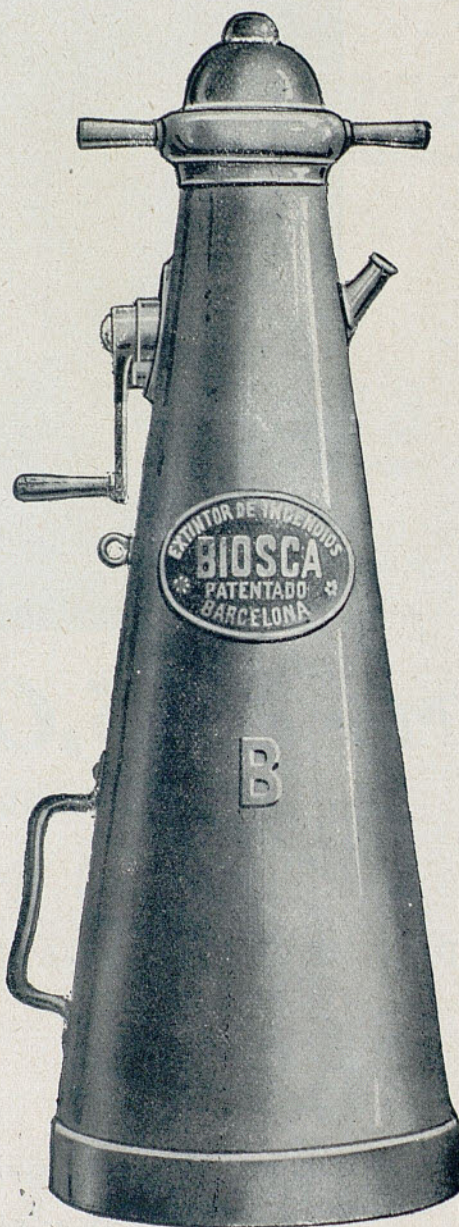
Aparato Modelo B de 10 litros de cabida, lanza el líquido extintor a 15 metros de distancia
