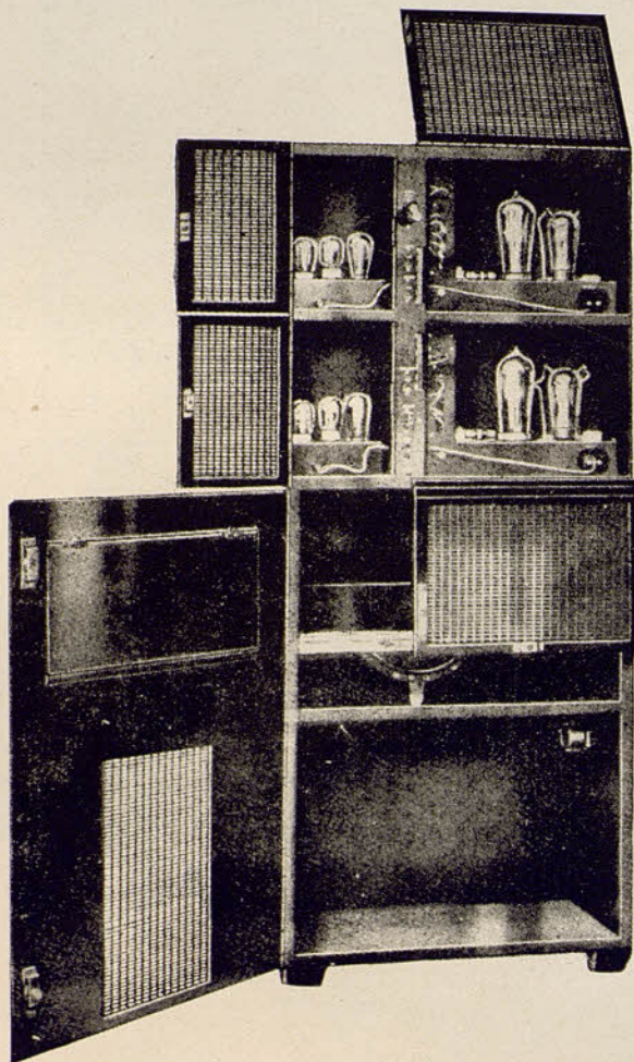
Doble amplificador abricado por la casa Philips Lamps, Ltd.
