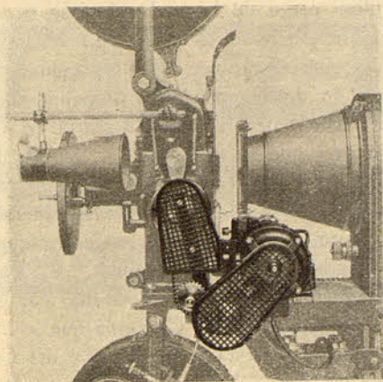
Crono HAHN II lado de la transmisión, con dispositivo sonoro tipo C
