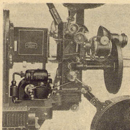
Crono ERNEMANN I con dispositivo sonoro tipo D
