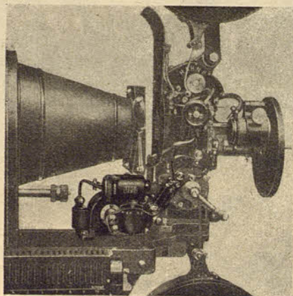
Crono HAHN II con dispositivo sonoro tipo D
