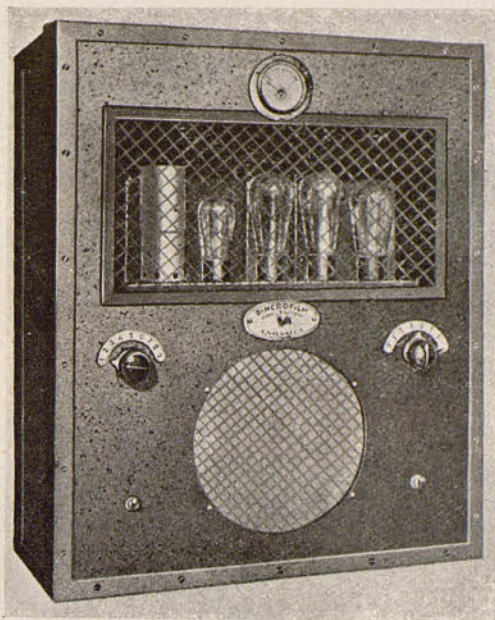
Amplificador de 6,5 vatios salida, provisto de: Altavoz piloto. Regulador de voltaje. Regulador de volumen de sonido
