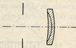
FIG. 12 OBJETIVO ACROMÁTICO SIMPLE
