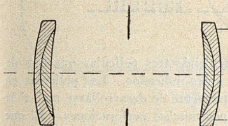
FIG. 13 OBJETIVO RECTILÍNEO O APLANÁTICO
